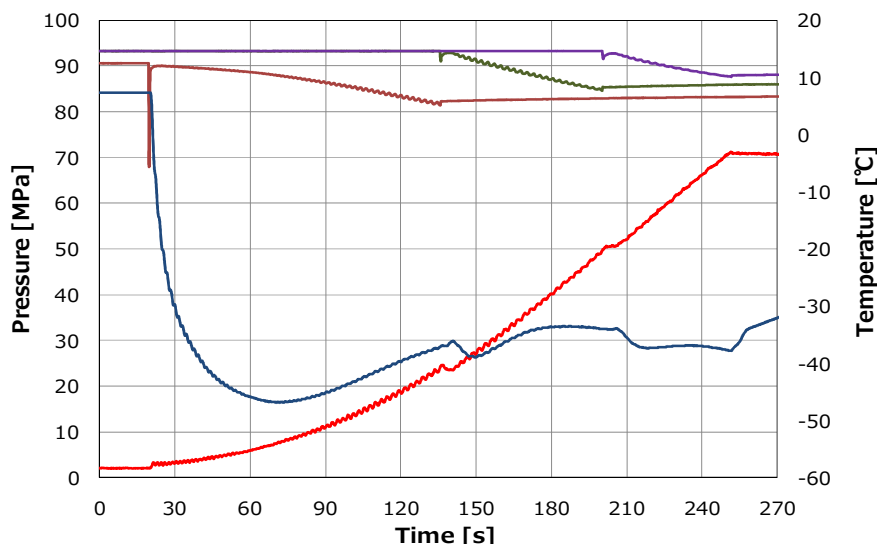
昇圧率制御充填試験
